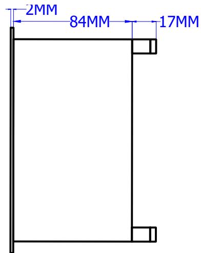
側視尺寸圖
